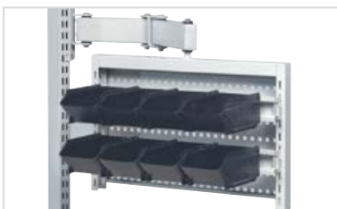
Drehbarer Universalhalter mit Lochblech M500, Aufhängeleiste M500 und 8 Kunststoffkästen ESD
