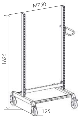
Basic-Wagen, Gestell
